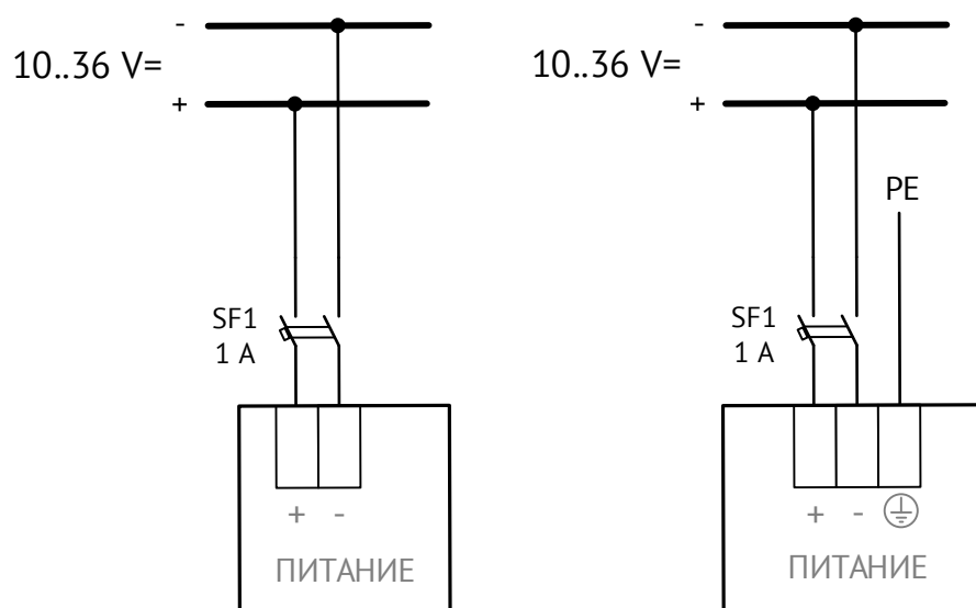
Рисунок 8.9. Схема подключения питания ЭНМИ-3/4м/7-24-1/2 (слева) и ЭНМИ-4м/4е-24-4 (справа)
