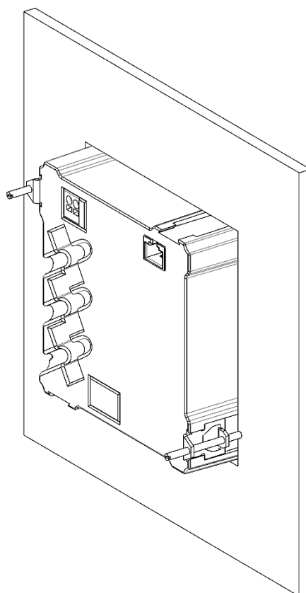
Рисунок 8.2. Модуль индикации ЭНМИ-Х-24-2, установленный в щит
